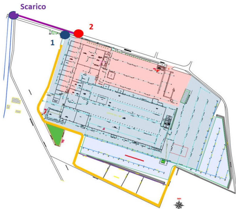
Figura 7 Layout ESISTENTE del reticolo fognario dello stabilimento:
